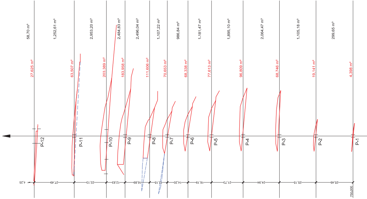
PERFIL TRANSVERSAL EJE DEL CANAL
