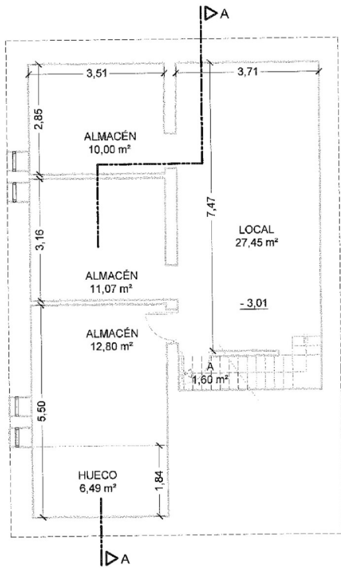
PLANTA SÓTANO
