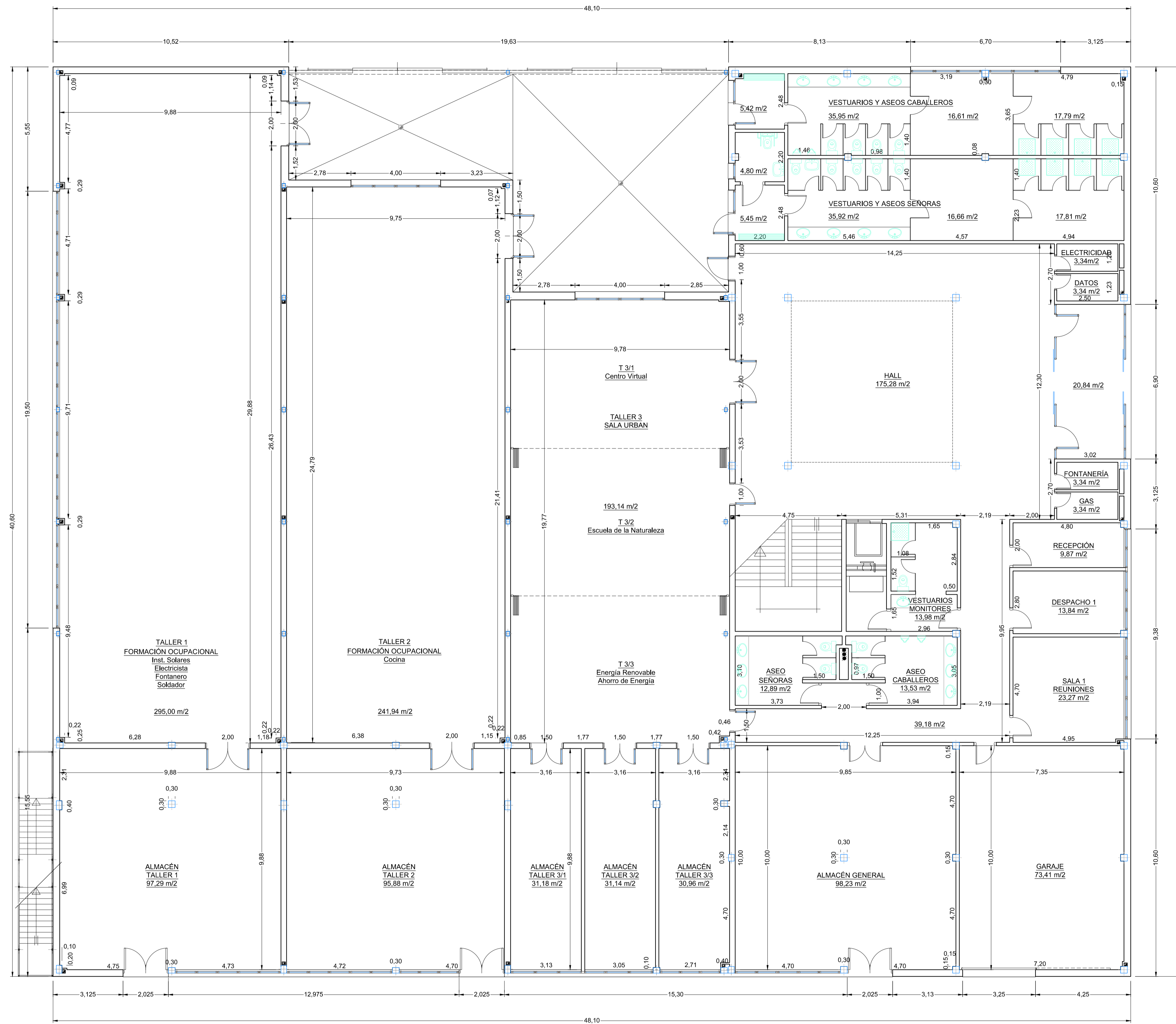
PLANTA BAJA COTAS Y SUPERFICIES
