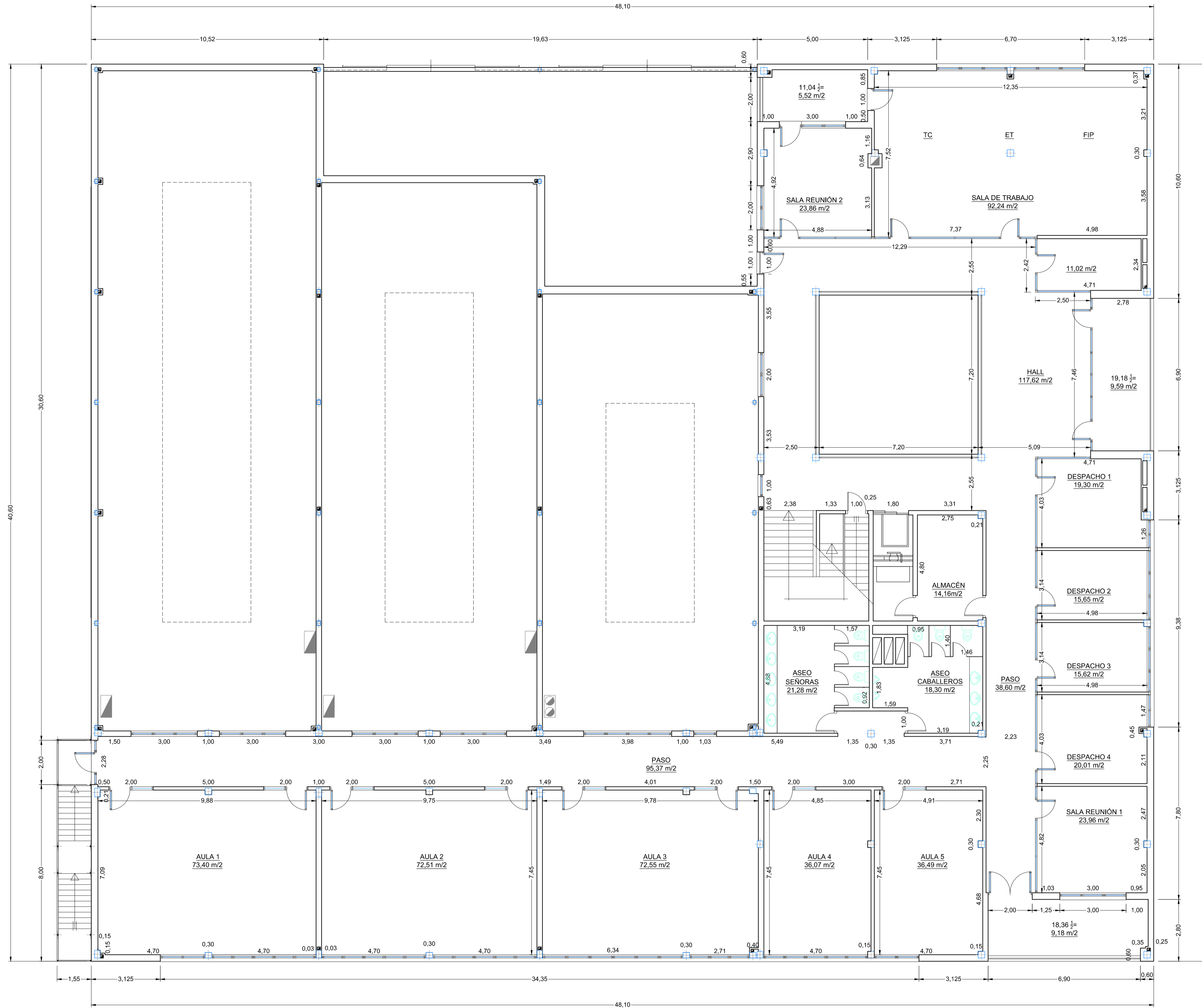
PLANTA PRIMERA COTAS Y SUPERFICIES
